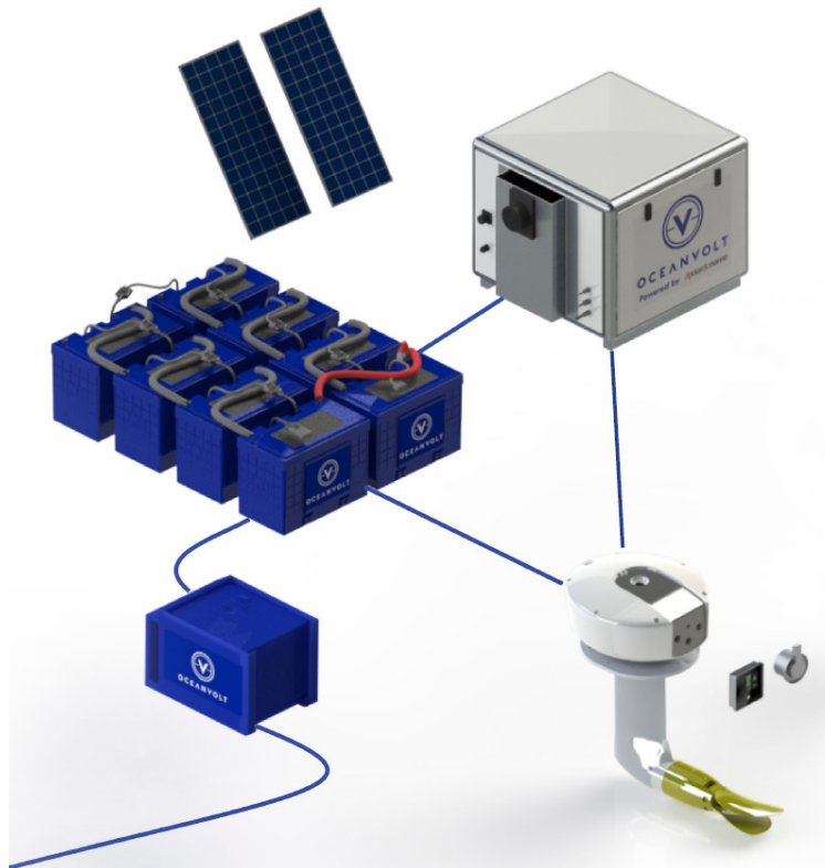
Arcona 380Z (Zero Emission) – komponenter for eldrift
